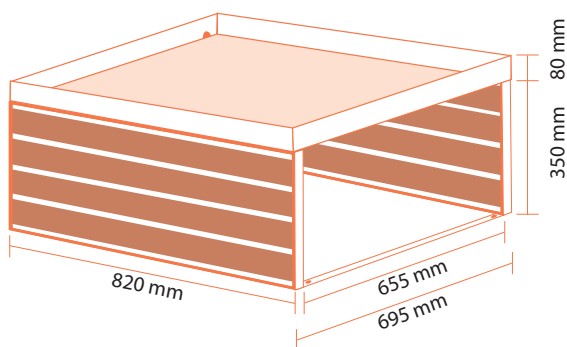
Mähroboter Garage Bloom | Art. Nr. 1101
