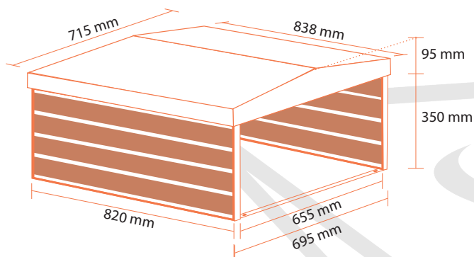
Mähroboter Garage Lodge | Art. Nr. 1100
